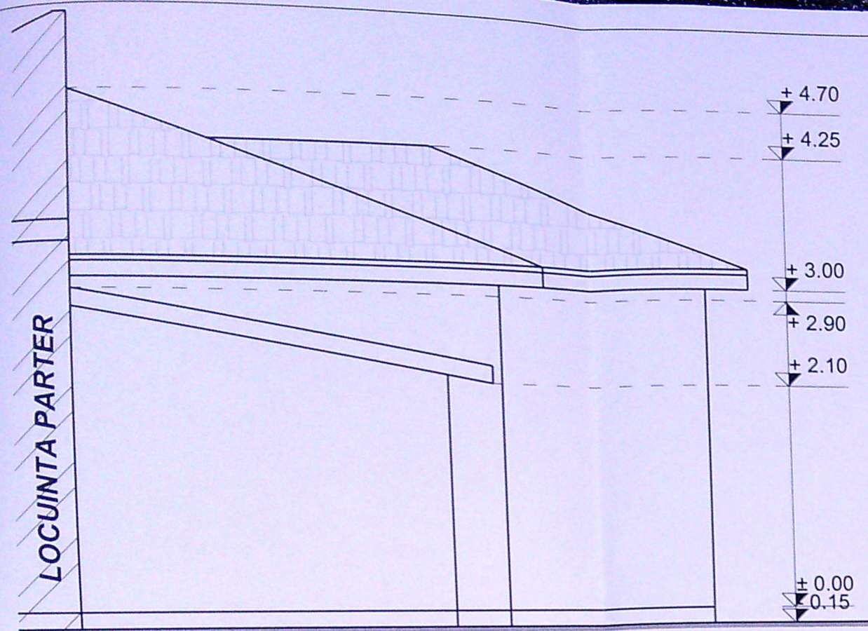
FATADA POSTERIOARA
